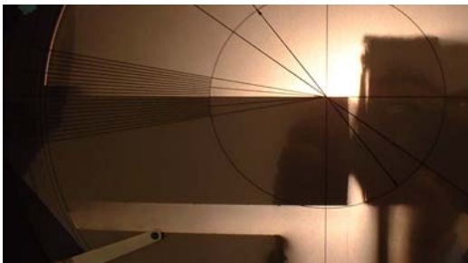
ST169: 0° top edge measurement
