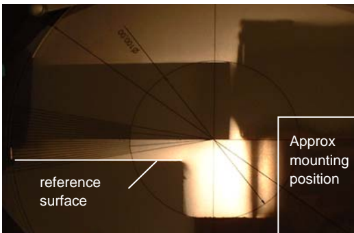
ST169: 0° bottom edge measurement
